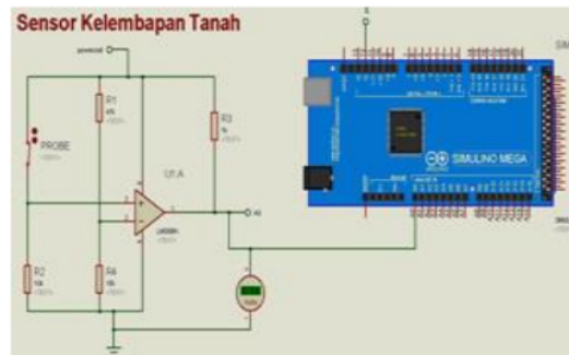
Gambar 4. Pengujian sensor kelembapan tanah
