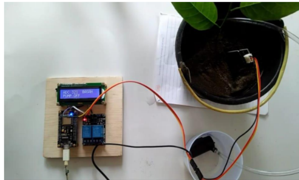
Gambar 7. proses pengujian Proses sistem
