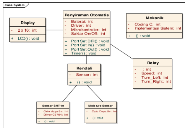
Gambar 2. Diagram Class sistem kerja Penyiram Tanaman
