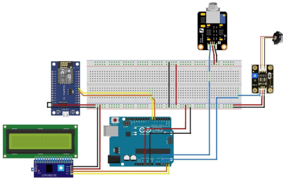
Gambar 3: Skema Rangkaian Smart Aquarium
