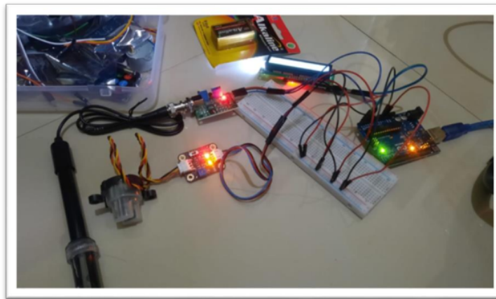
Gambar 4: Implementasi Perangkat Keras
