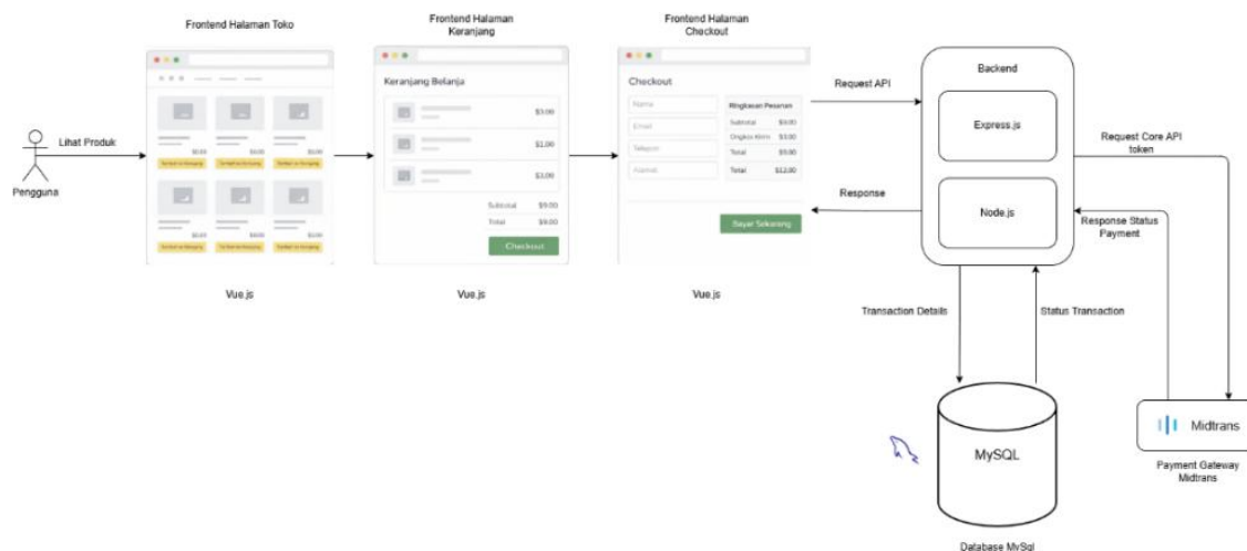
Gambar 2. Alur Arsitektur Sistem Pembayaran
