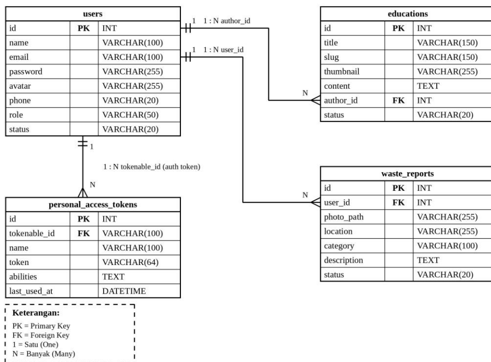
Gambar 2. Struktur Tabel dan Relasi Basis Data
