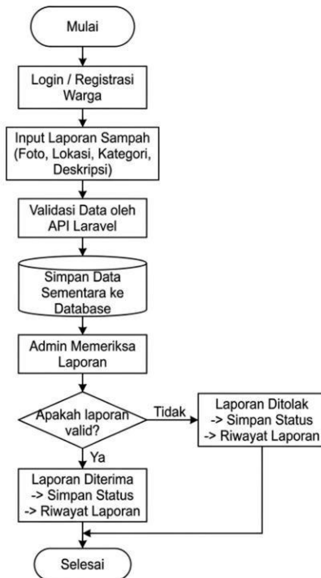
Gambar 3. Alur Pelaporan dan Verifikasi Sampah
