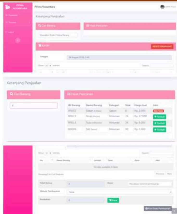
Gambar 10. Halaman Transaksi
