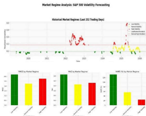
Gambar 11. Visualisasi Rezim Volatilitas Historis S&P 500
