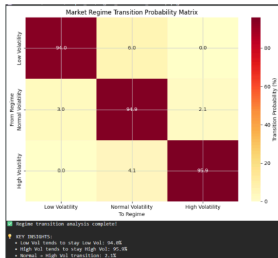
Gambar 10. Matriks Transisi Rezim Volatilitas
