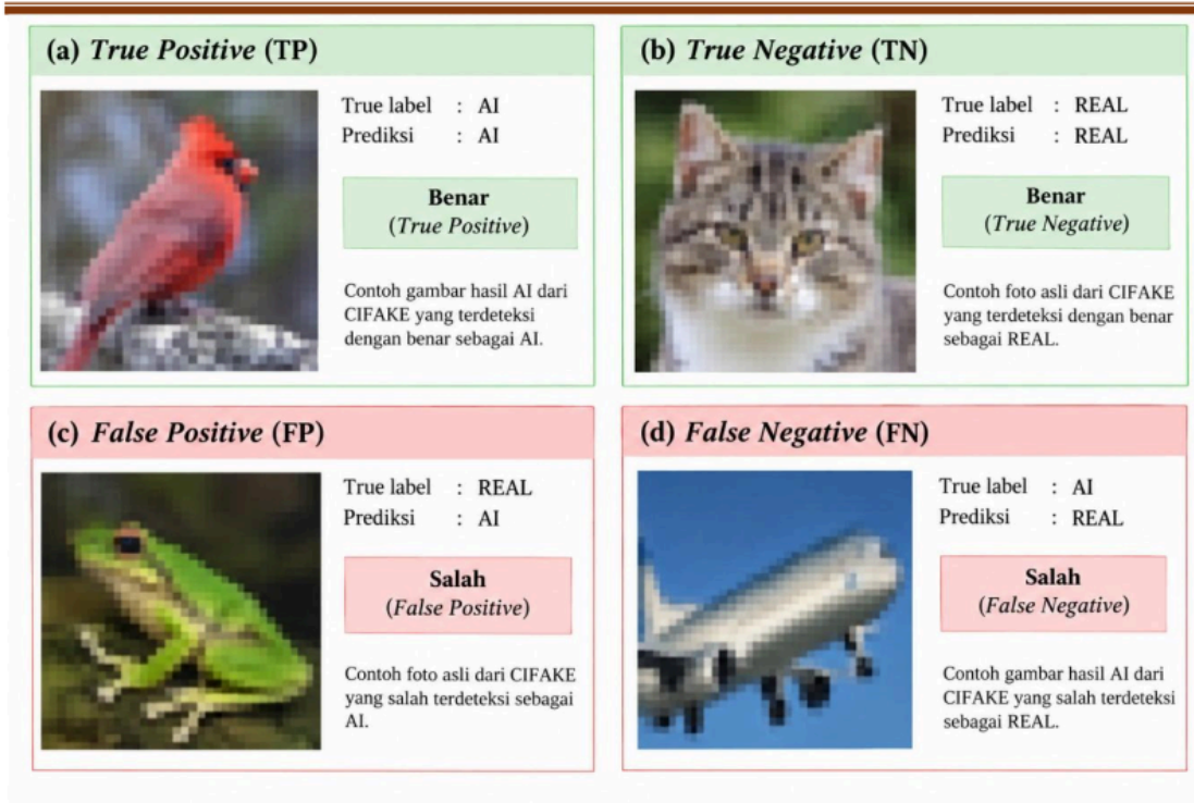
Gambar 5. Contoh Hasil Klasifikasi True Positive (TP) , True Negative (TN) , False Positive (FP) , dan False Negative (FN)
