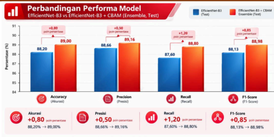
Gambar 3. Perbandingan metrik ensemble pada data uji terpisah
