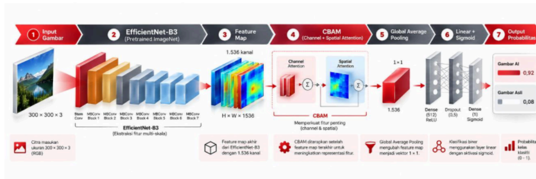
Gambar 2. Arsitektur EfficientNet-B3 dengan CBAM
