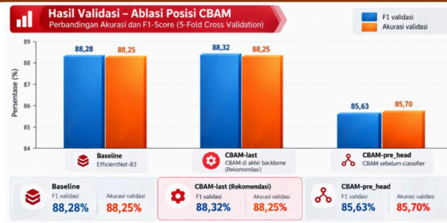
Gambar 6. Perbandingan hasil ablasi posisi CBAM
