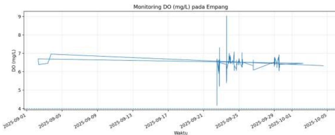
Gambar 5. Grafik Hasil Monitoring Oksigen Terlarut
