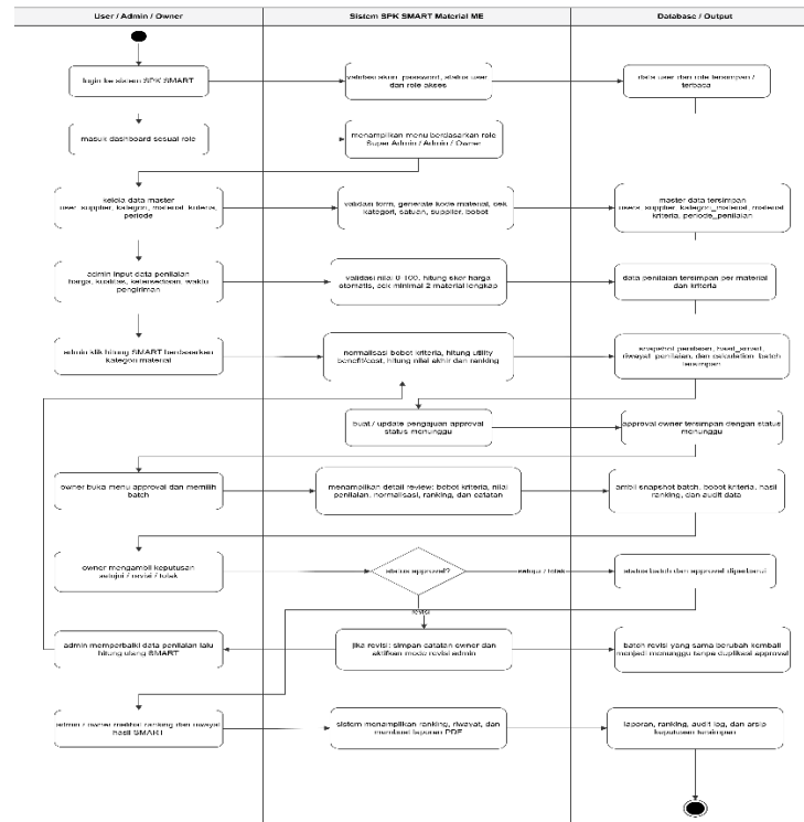
Gambar 1. Sistem Usulan
