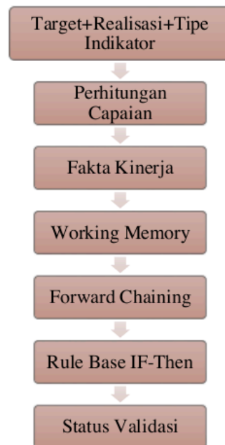
Gambar 3. Model Inferensi Dua Tahap
