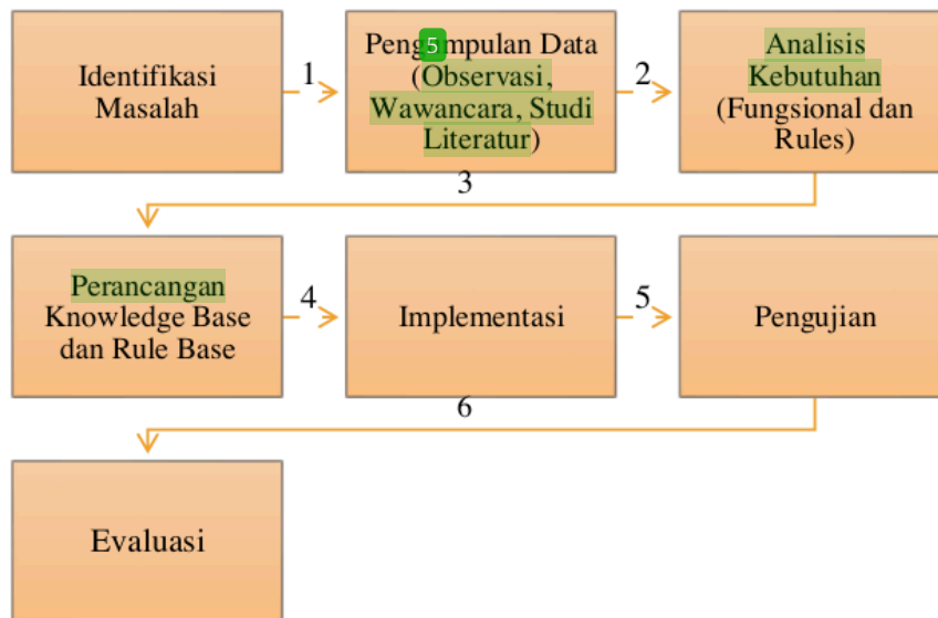
Gambar 1. Tahapan Penelitian
