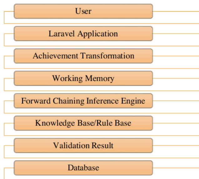
Gambar 2. Arsitektur Model
