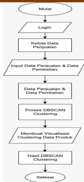
Gambar 2. Analisis Sistem Usulan
