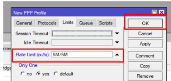
Gambar 7. Limit Kecepatan pada Masing-Masing Profil
