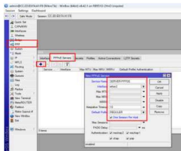
Gambar 9. Konfigurasi PPPoE Server
