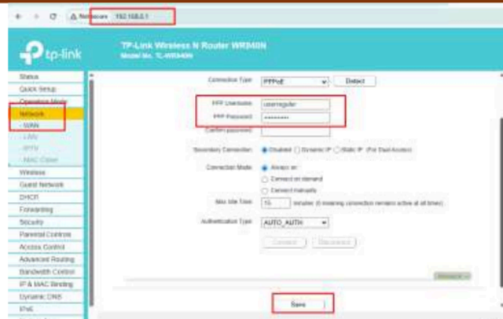
Gambar 14. Setting PPPoE Client pada Router
