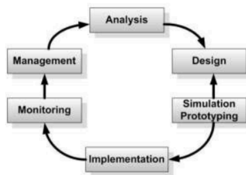
Gambar 1. Tahapan NDLC
