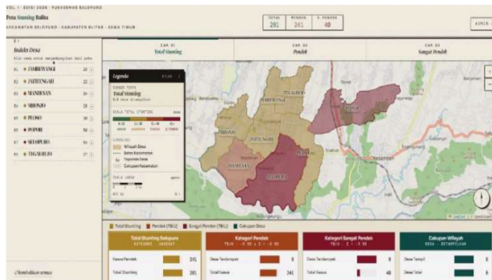
Gambar 5. WebGIS Stunting
