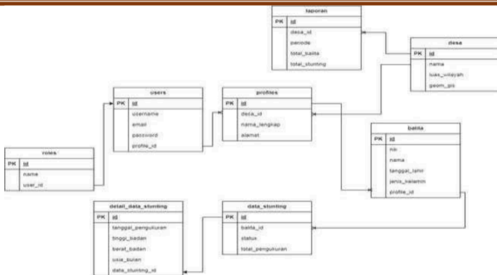
Gambar 3. ERD
