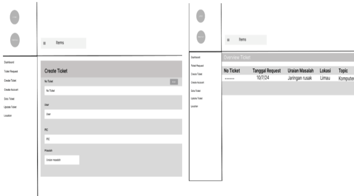
Gambar 6. Wireframe Sistem
