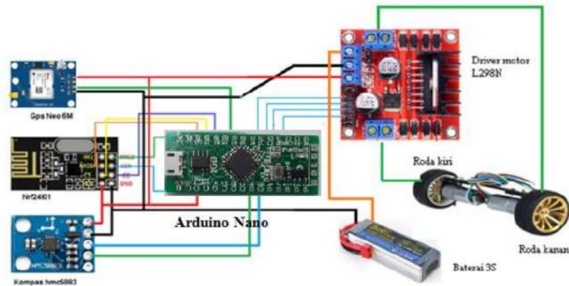
Gambar 4. Rancangan Perangkat Elektronik
