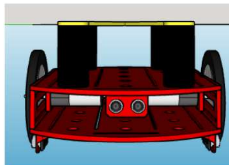
Gambar 6. Desain mekanik robot tampak depan
